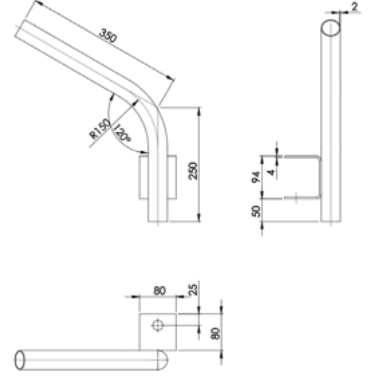
Armatür Boru
